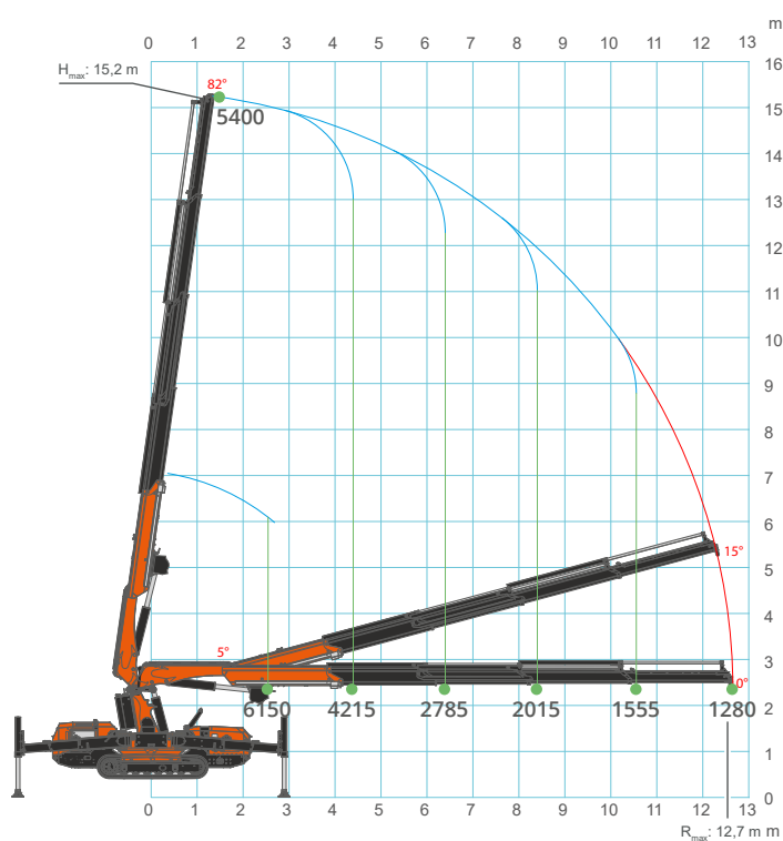
Hoofdmast
