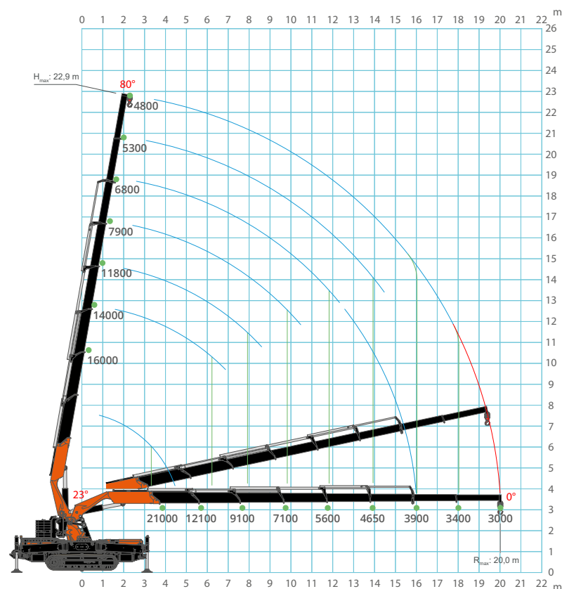
Hoofdmast
