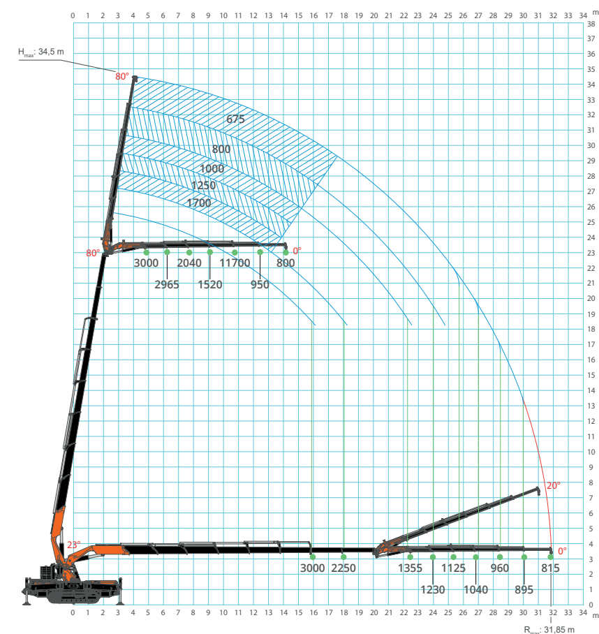
Hydraulische jib
